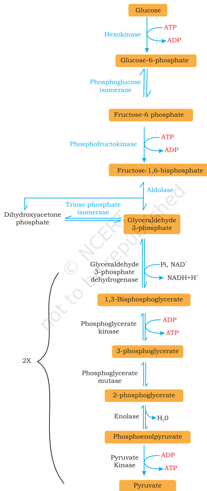
Fig. 5.4: Glycolysis
